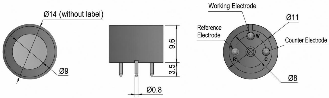
SX-GO2TMA Mini Lead-Free Oxygen Sensor Dimensions
